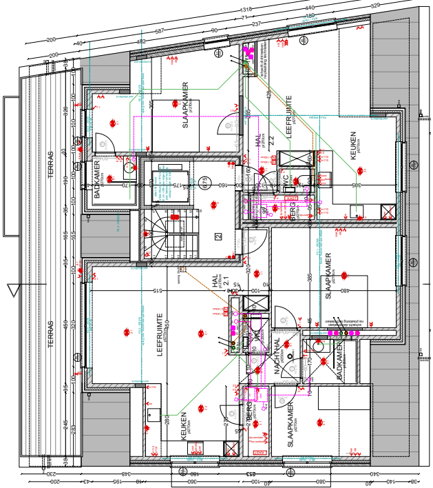
NIVEAU +2
