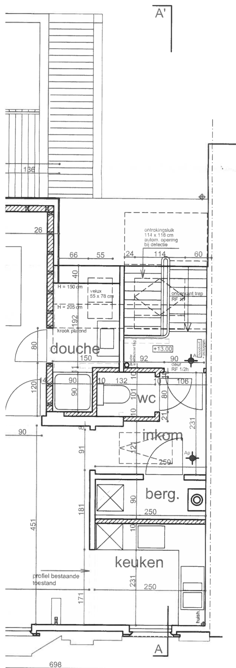
verdieping 4
