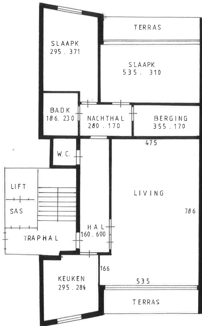
VERDIEPING 2
