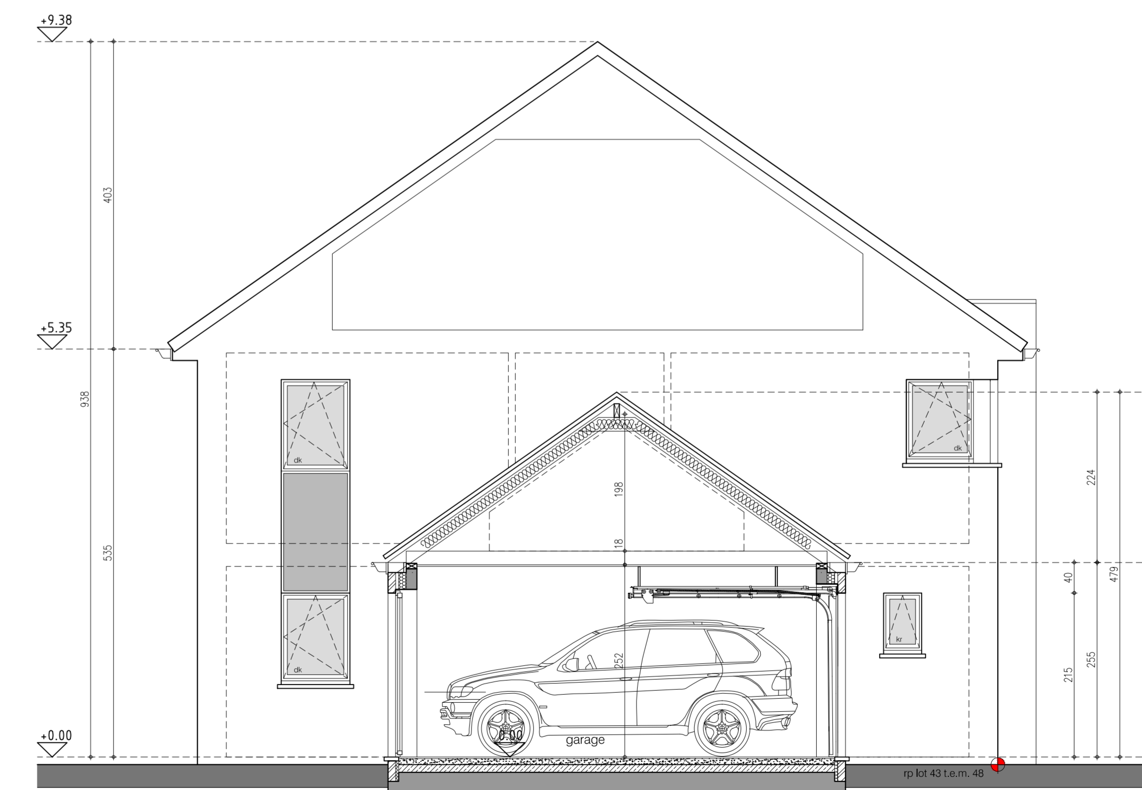
zijgevel lot 46
