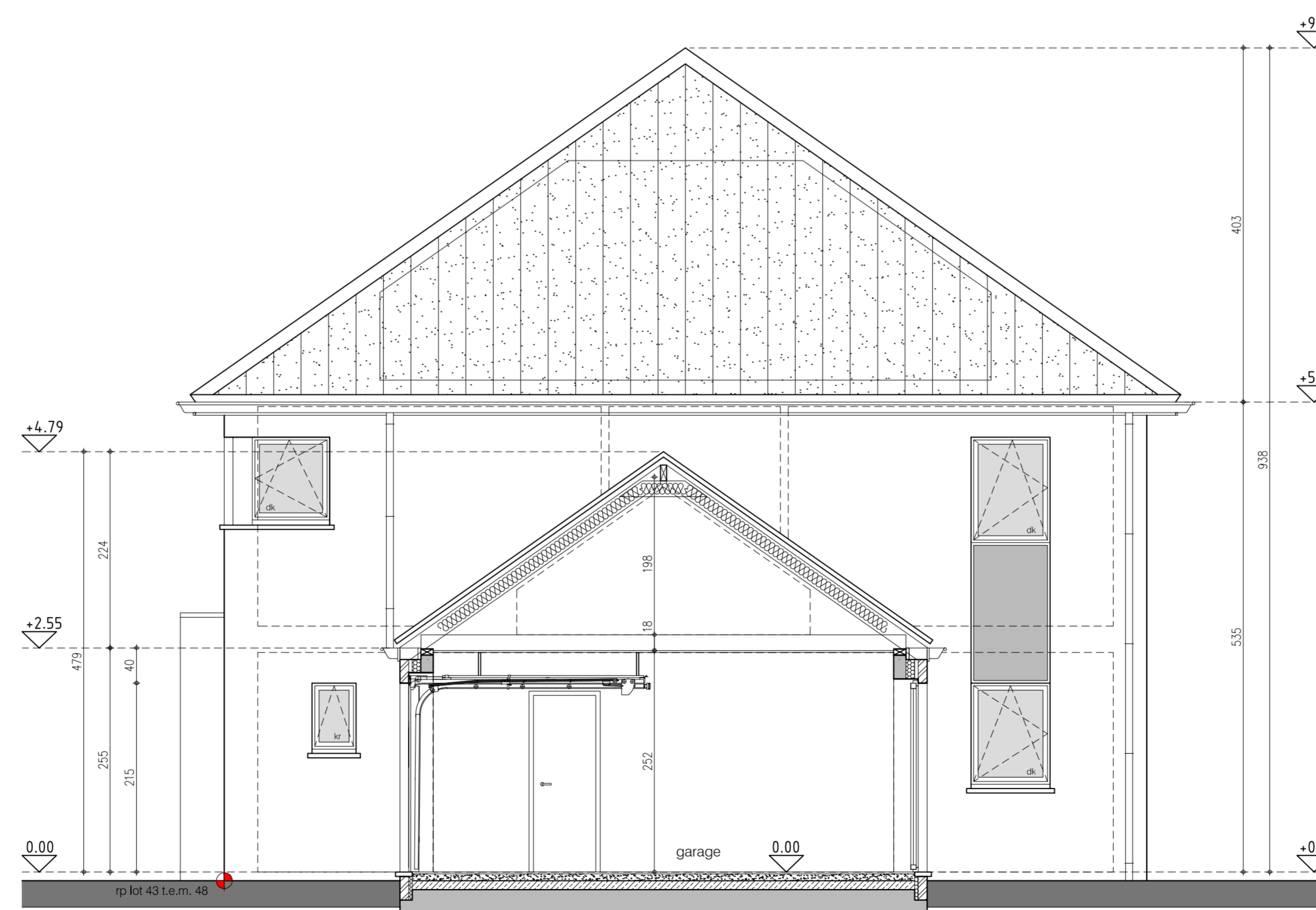
zijgevel lot 47
