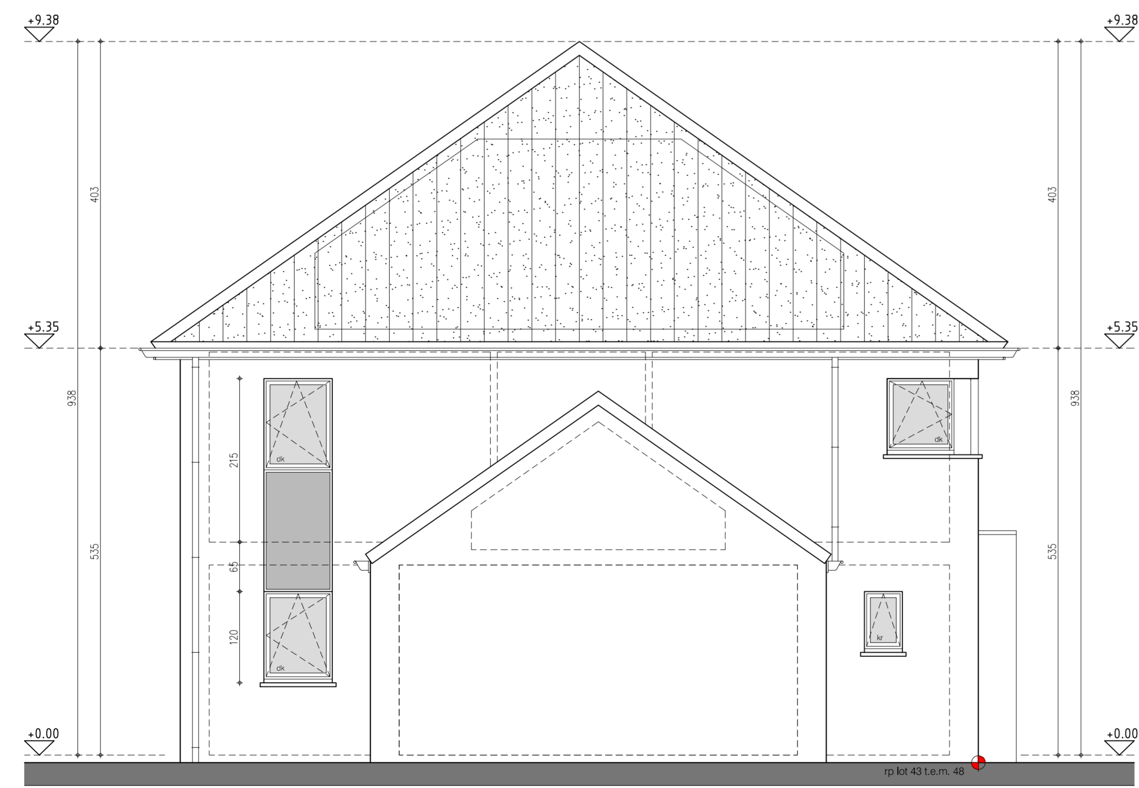
zijgevel lot 48
