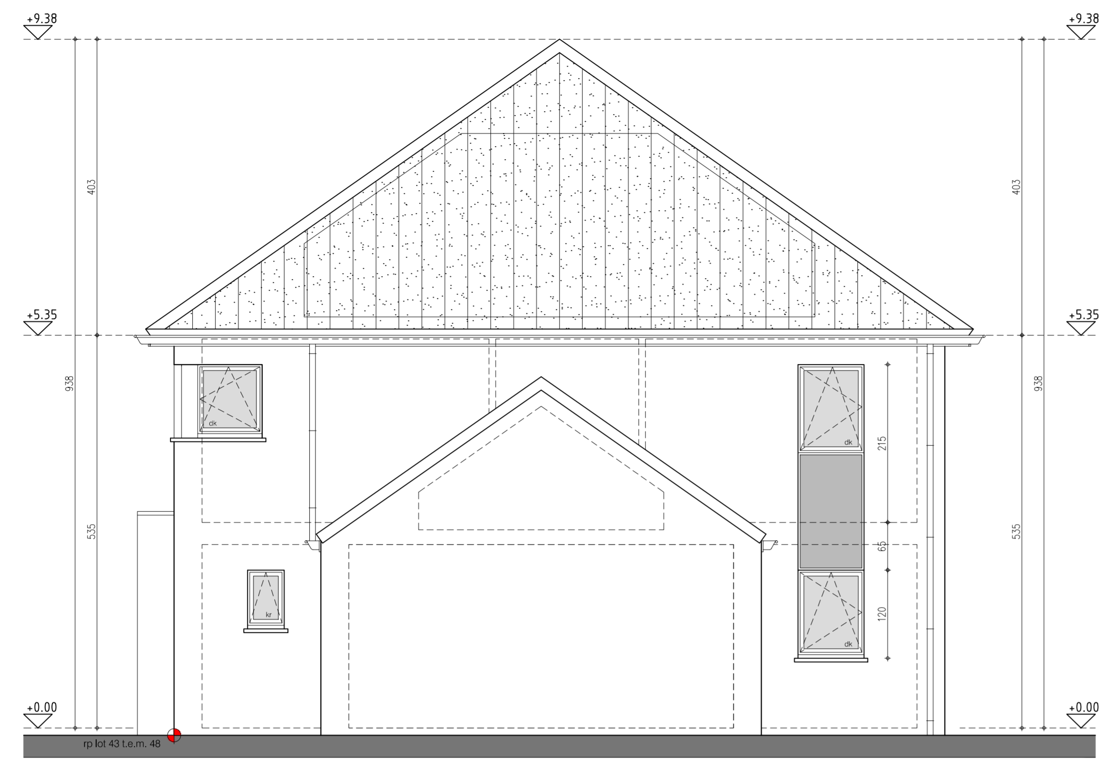
zijgevel lot 43
