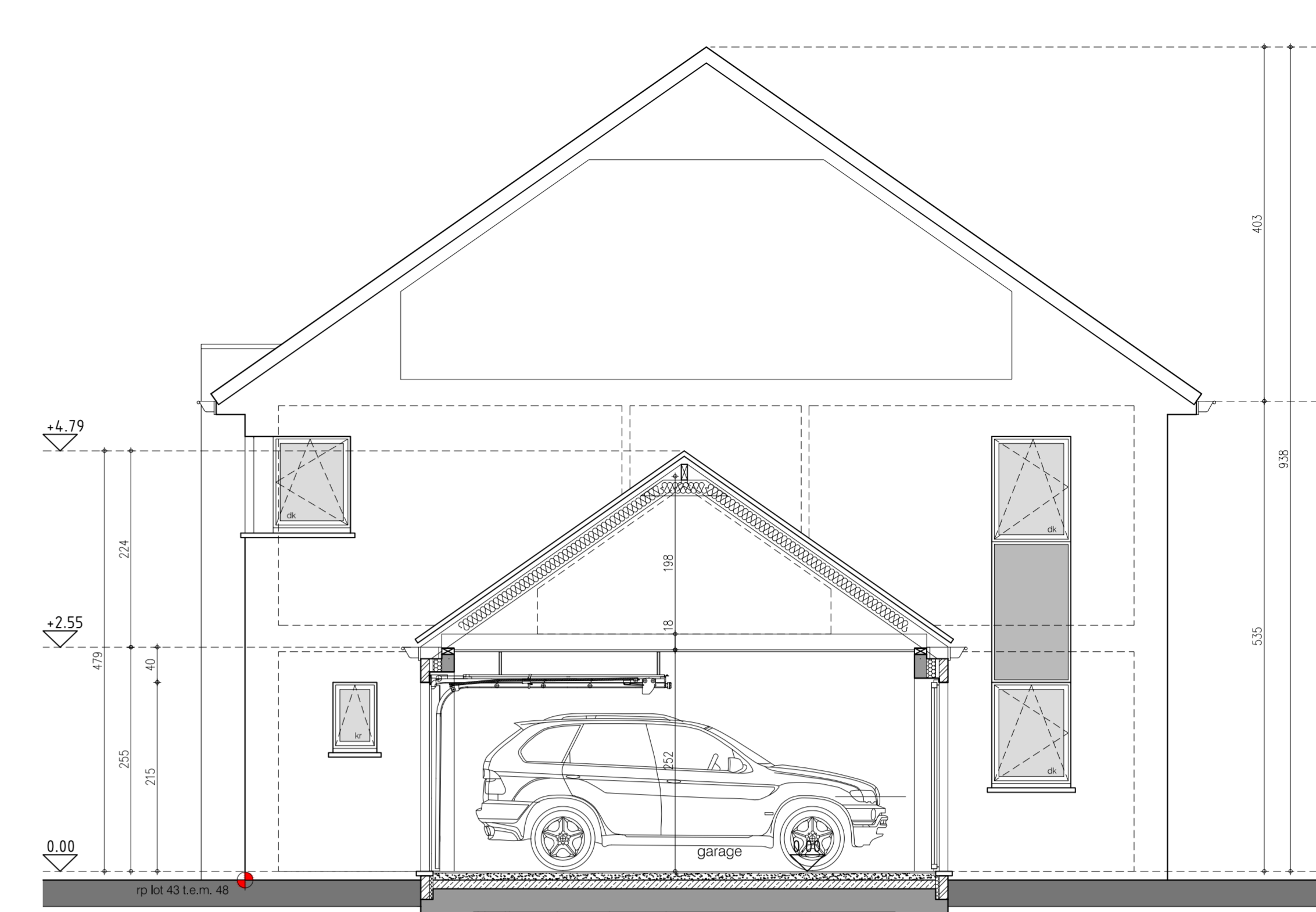
zijgevel lot 45
