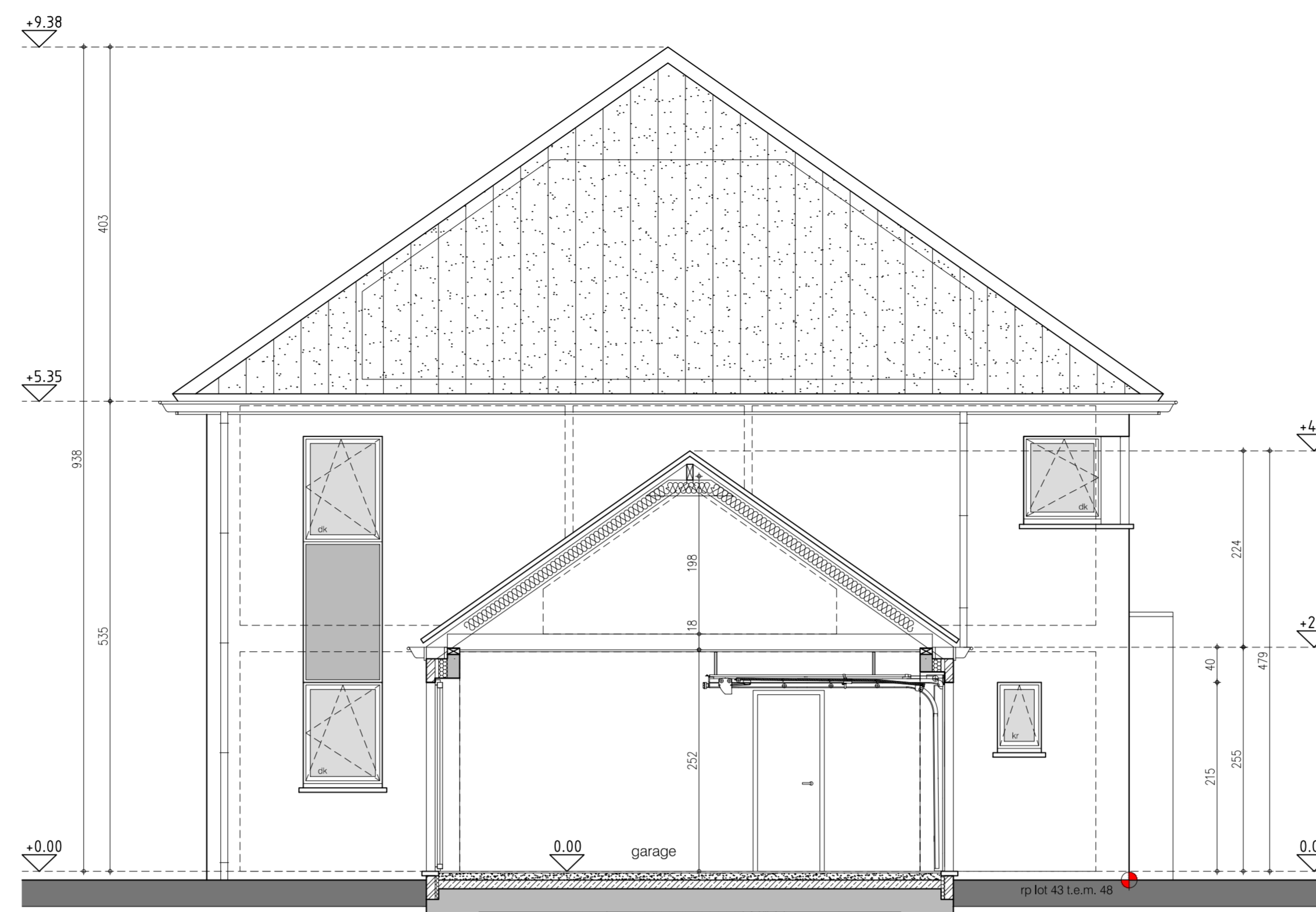
zijgevel lot 44
