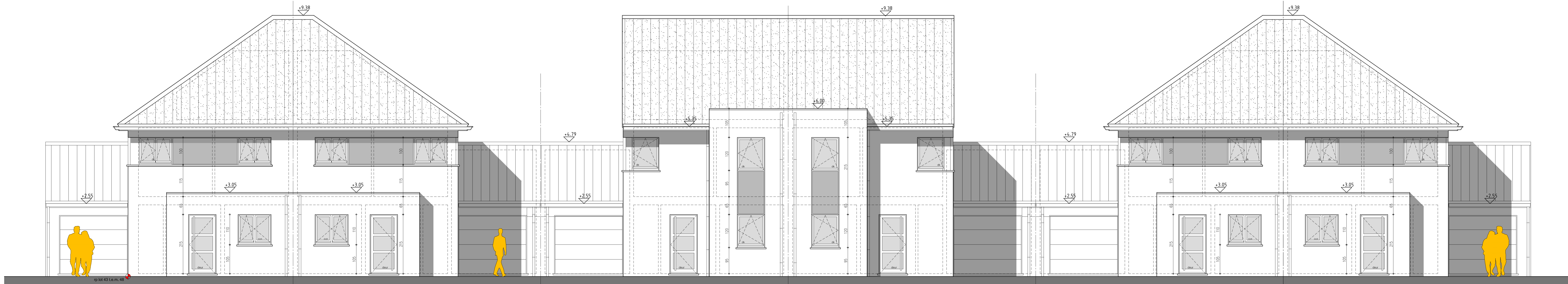
voorgevel lot 48
