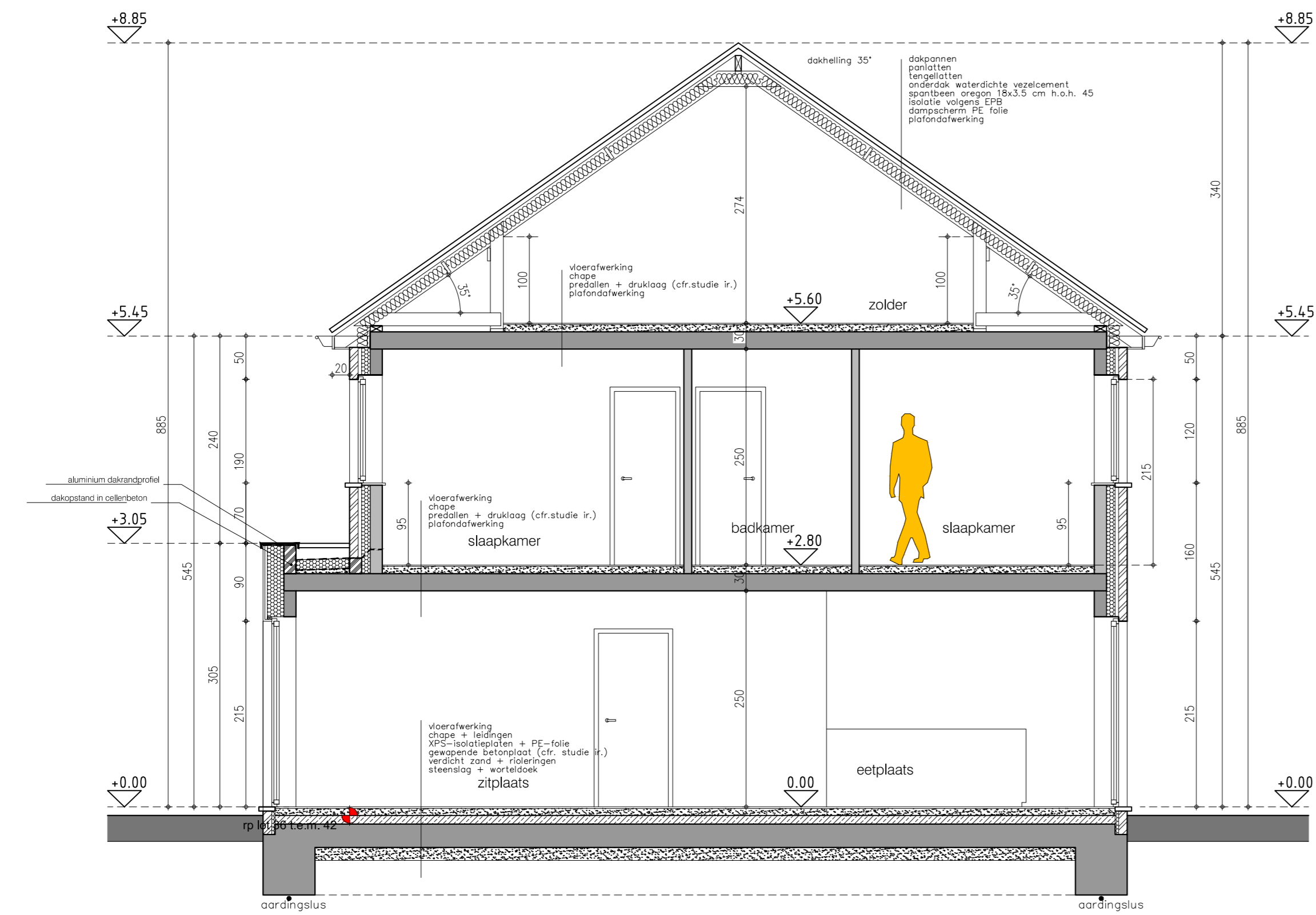
doorsnede D1 - D1 lot 38 en 41 typesnede lot 36 - 42
