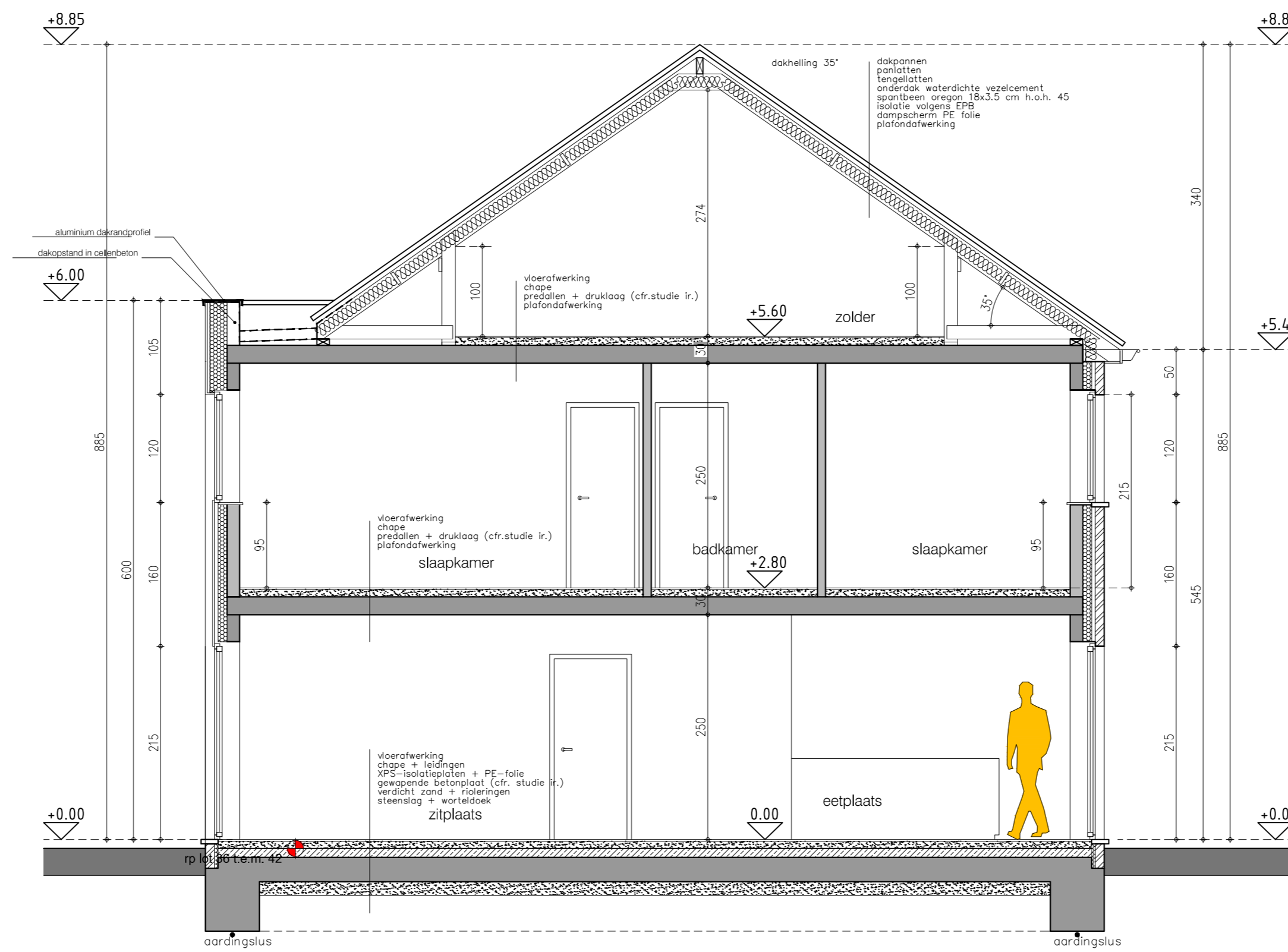
doorsnede D2 - D2 lot 40
