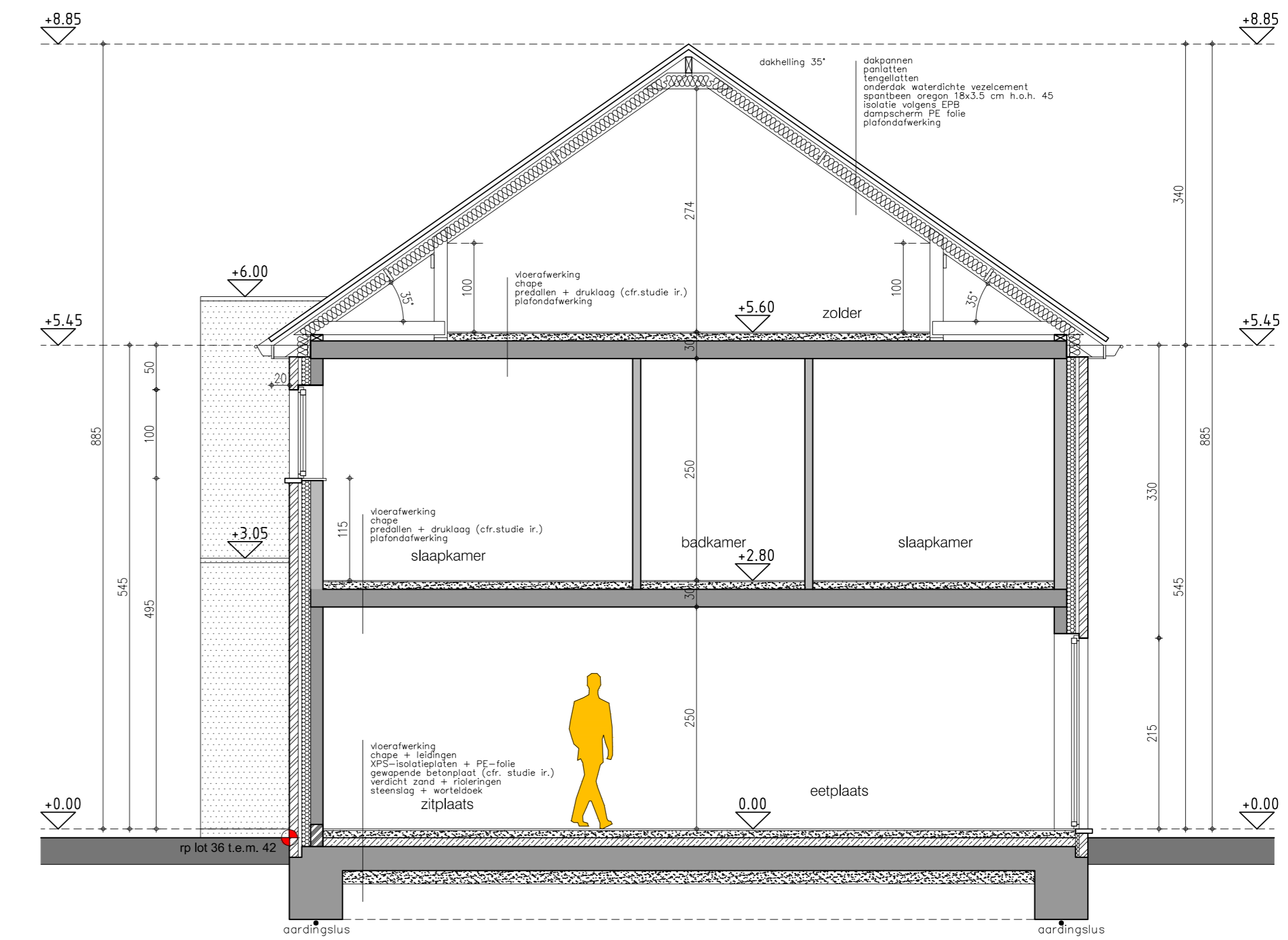
doorsnede D3 - D3 lot 37 en 39 typesnede lot 36 - 42
