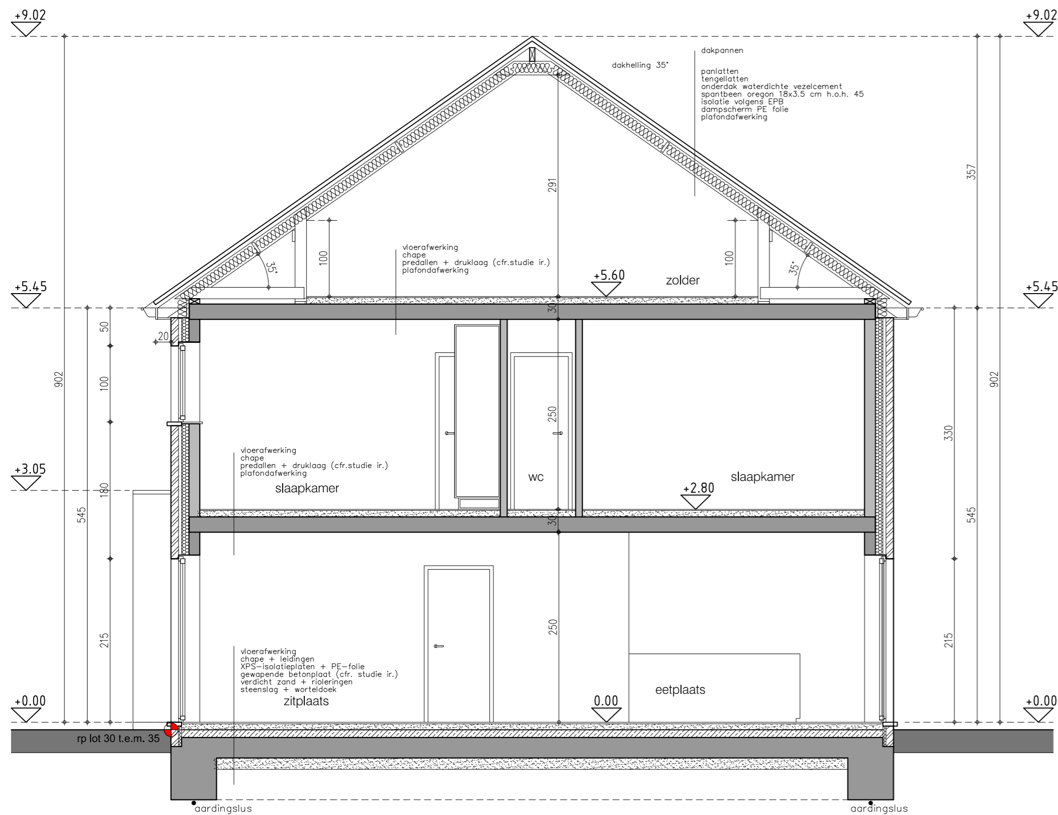
doorsnede C1 - C1 lot 31 en 33 typesnede lot 30 - 35
