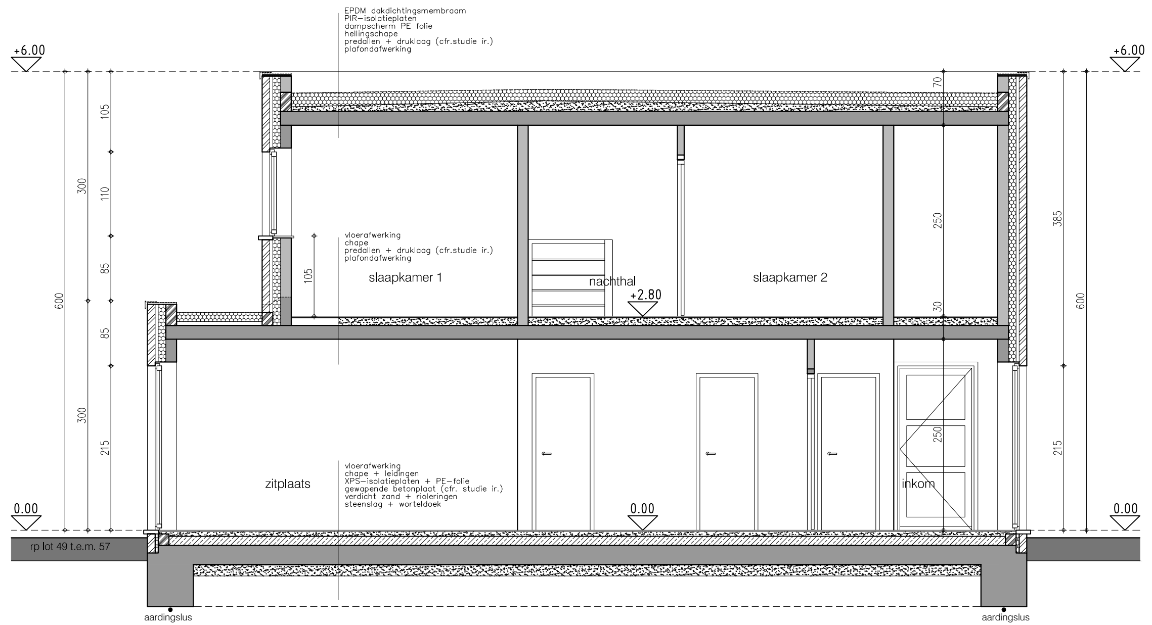
doorsnede G1 - doorsnede lot 1 en 2 type snede voor lot 3
