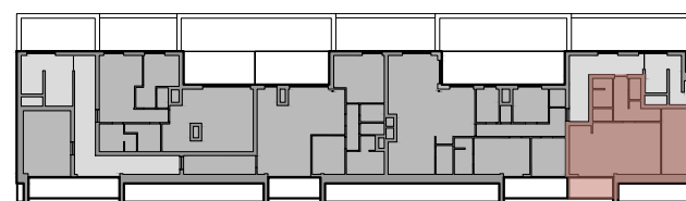
Grondplan niveau +3
